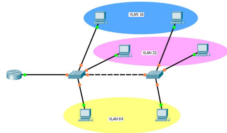
Figura 1. Topología.
